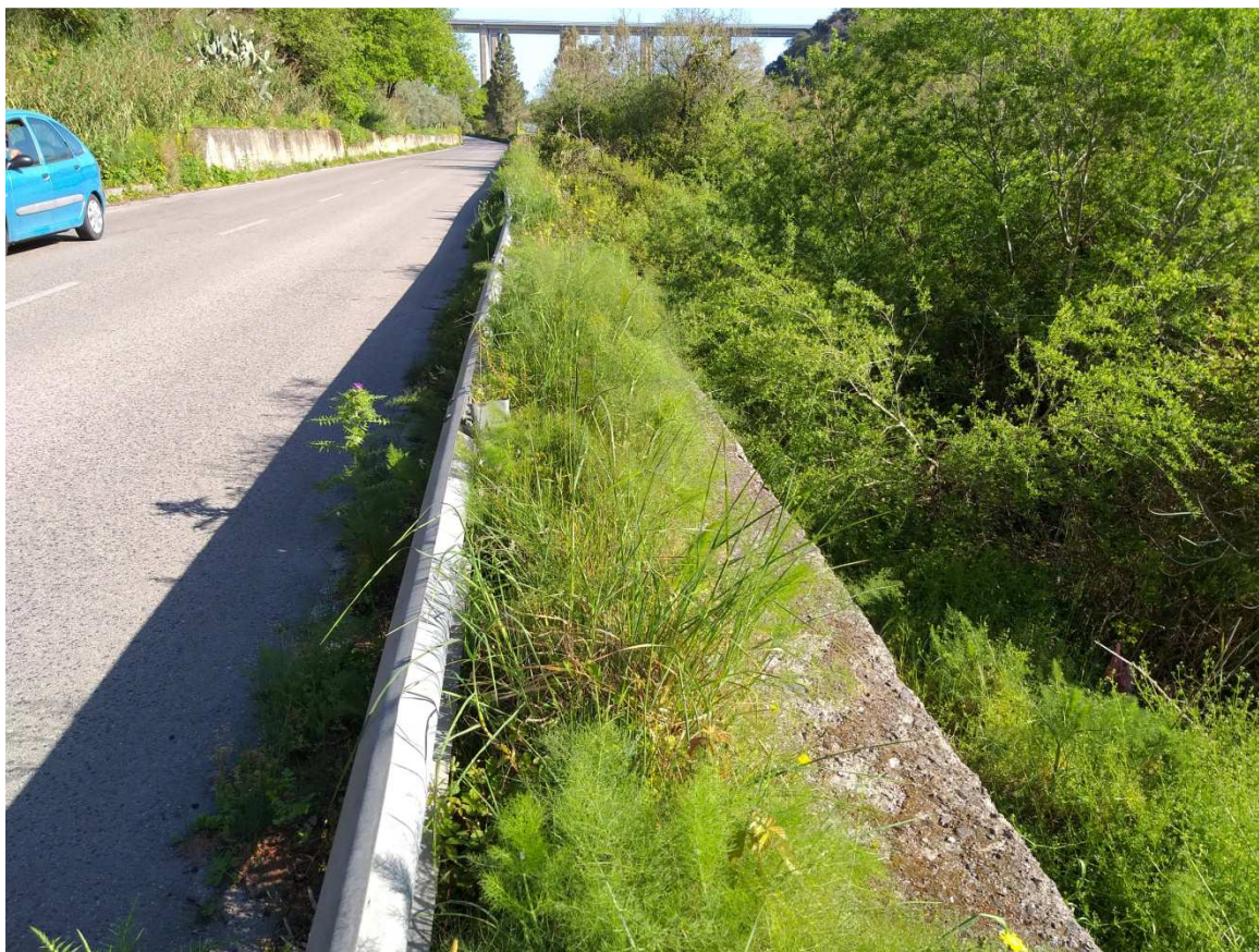
Foto N° 3: Tratto di barriera metallica di sicurezza da sostituire con barriera metallica di sicurezza del tipo H2 su manufatto, da posizionare sul muro d'argine.
