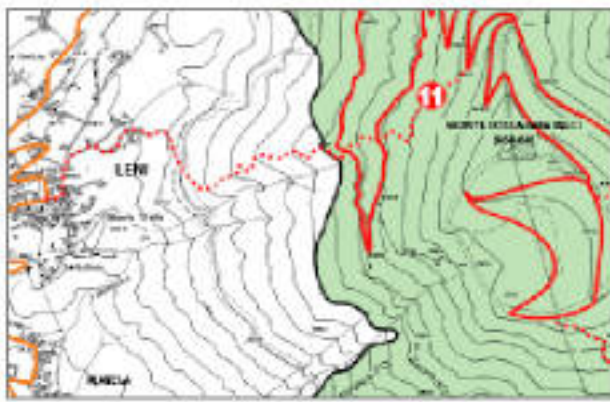
Stralcio Planimetrico
